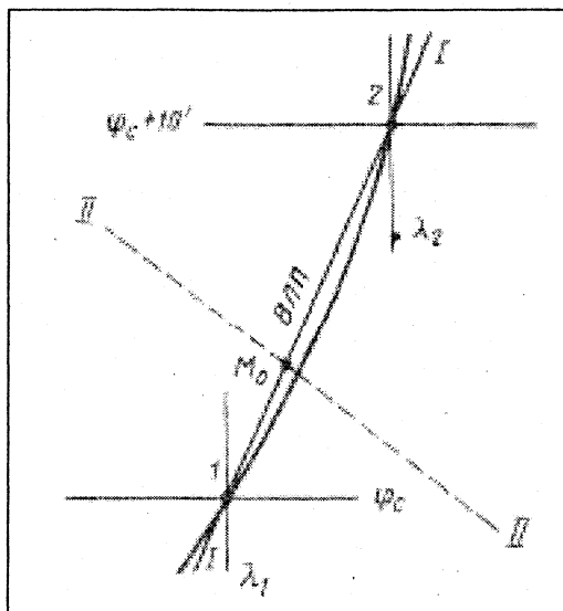
I-I — линия положения, построенная методом Сомнера.
