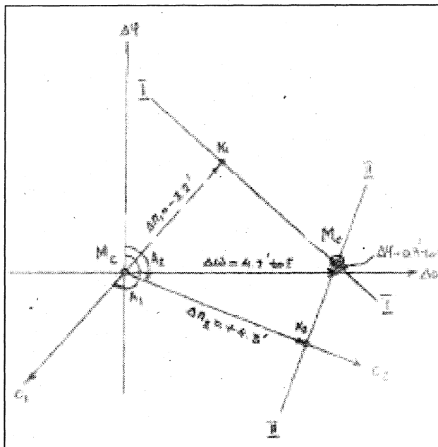
Определение места судна методом Сент-Илера.
